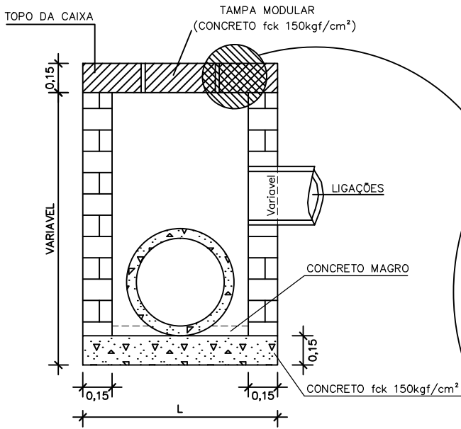
CORTE A-A
