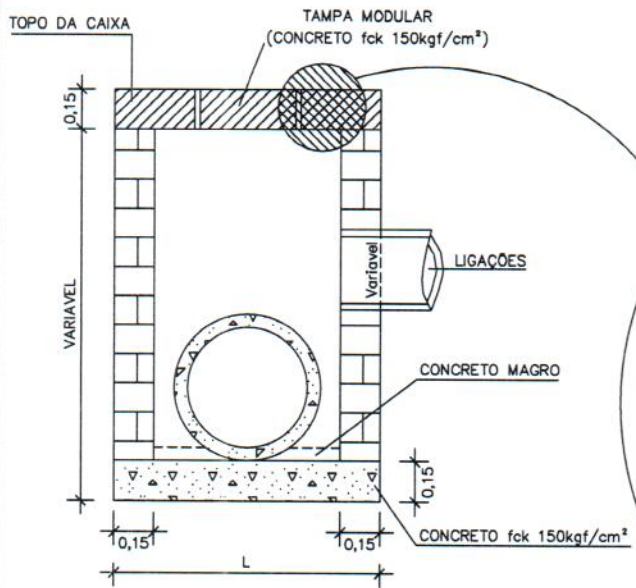
CORTE A-A
