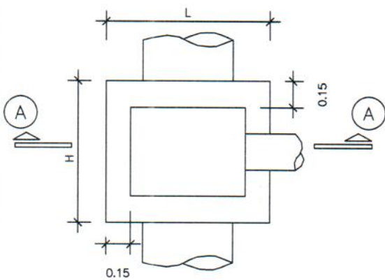
PLANTA
