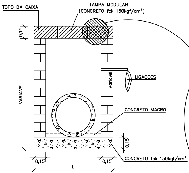
CORTE A-A
