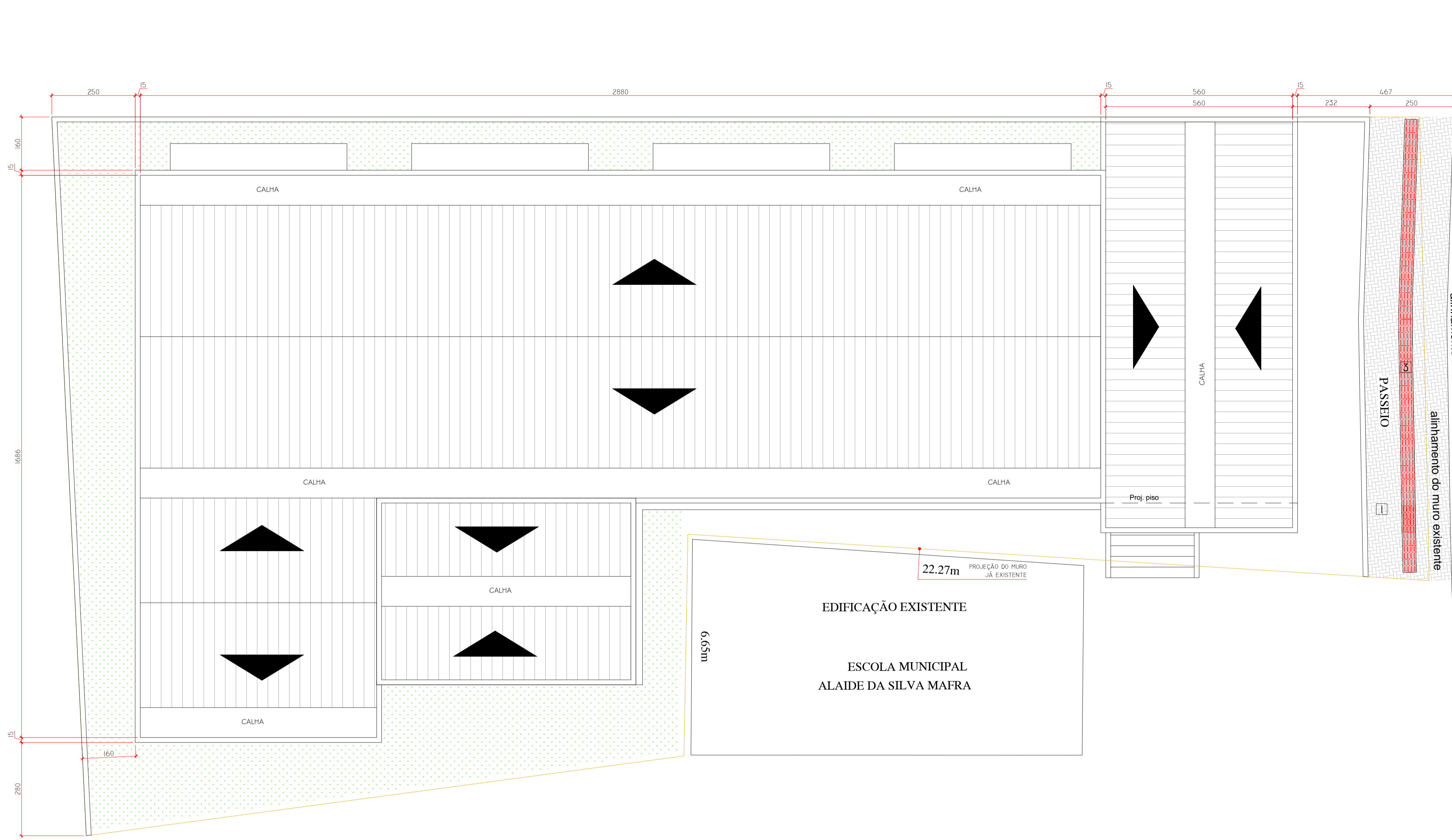
02 PLANTA DE COBERTURA Esc. 1/75
