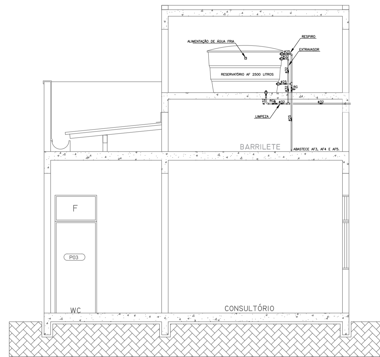
08 CORTE AA Esc. 1/50
