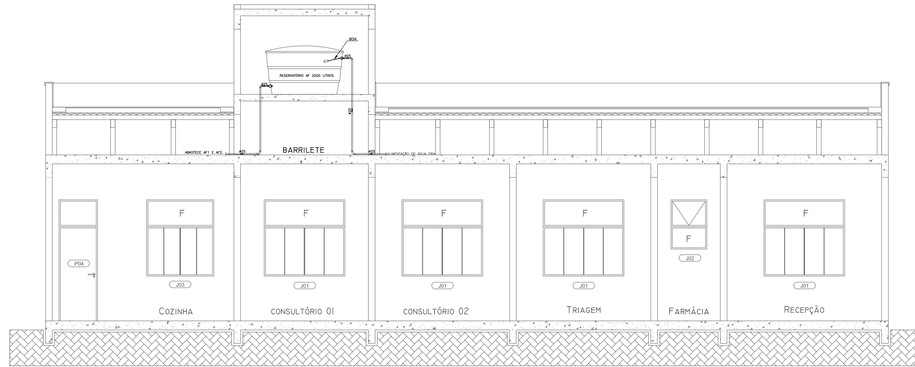
09 CORTE BB Esc. 1/50
